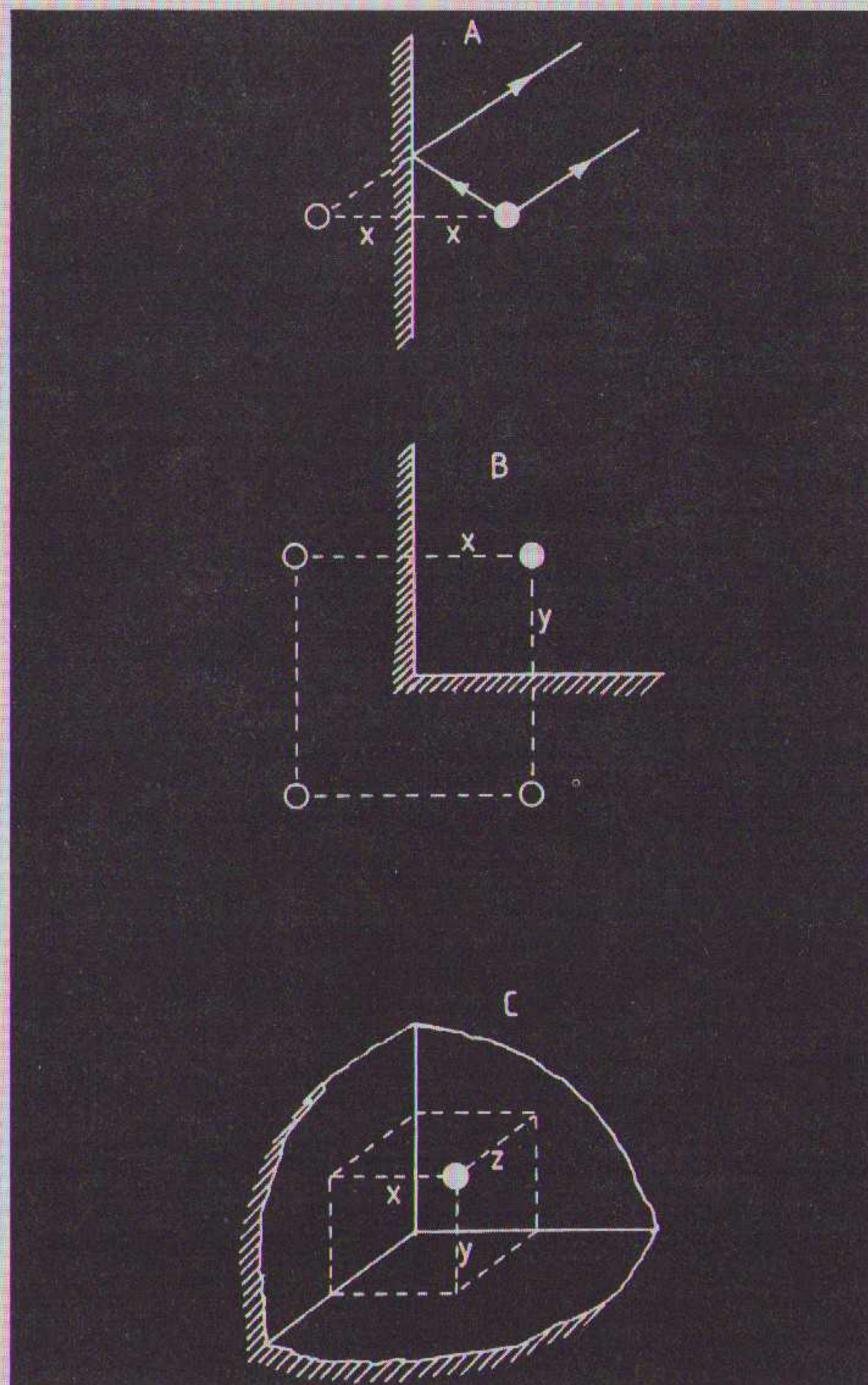
Fig. 43. Een geluidsbron (zwarte bol) in de nabijheid van één grensvlak (A), twee grensvlakken (B) en drie grensvlakken (C). De witte bollen zijn spiegelbronnen.
